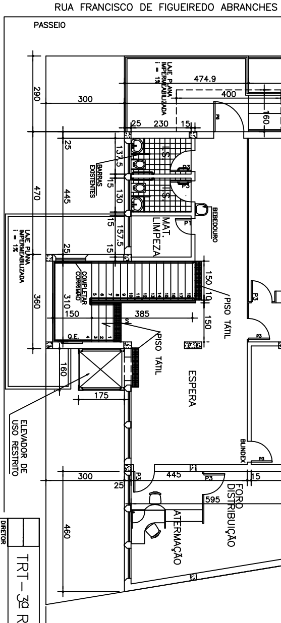
1º PAVIMENTO ESC.: 1:100 AREA: 238,60 m2
