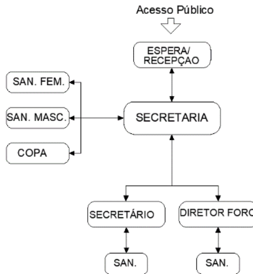
Figura 04 - Distribuição esquemática dos ambientes do Apoio à 1ª Instância Fonte: Secretaria de Engenharia
