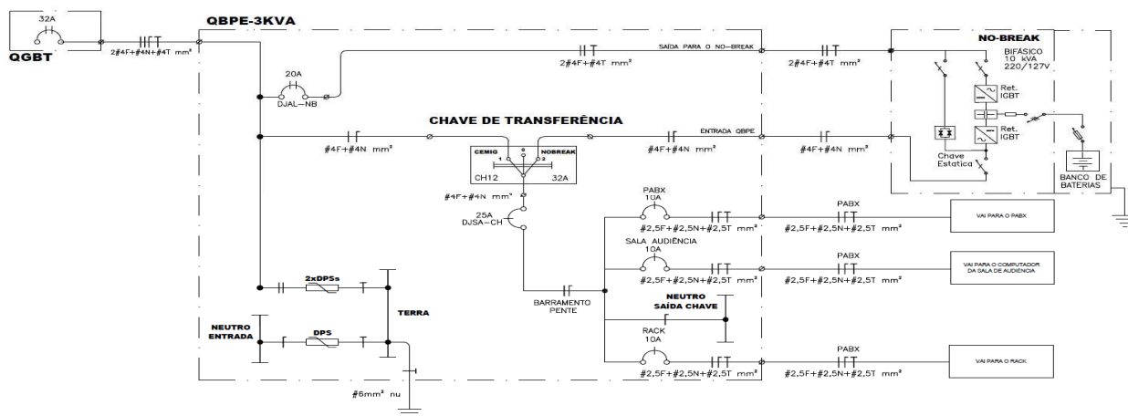
DIAGRAMA UNIFILAR QBPE - 3KVA
